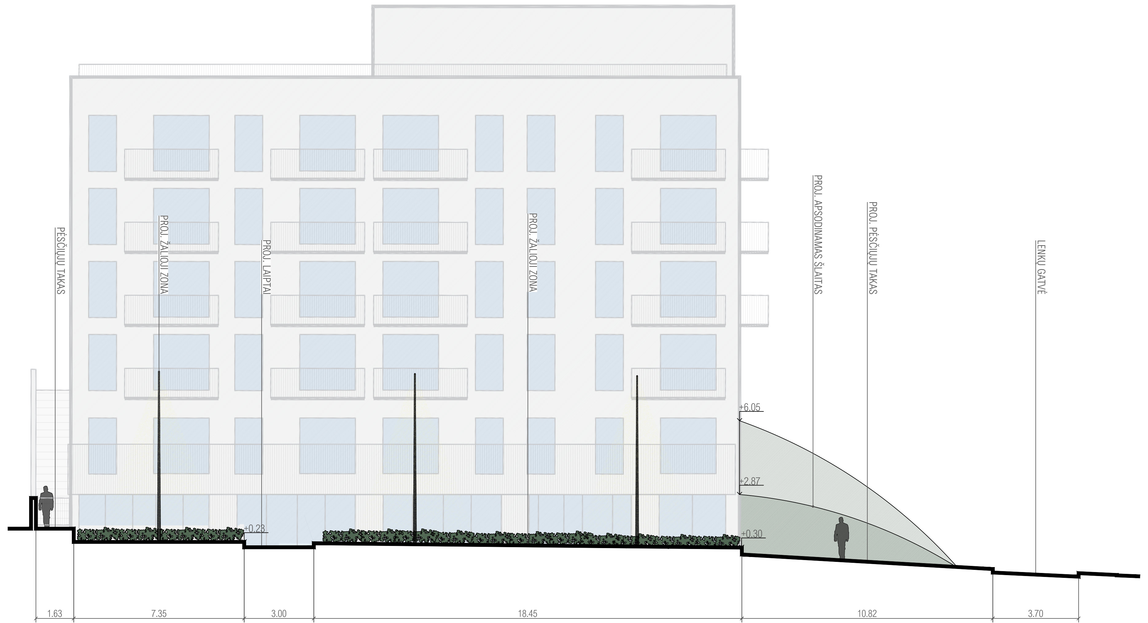
Pjūvis A-A
