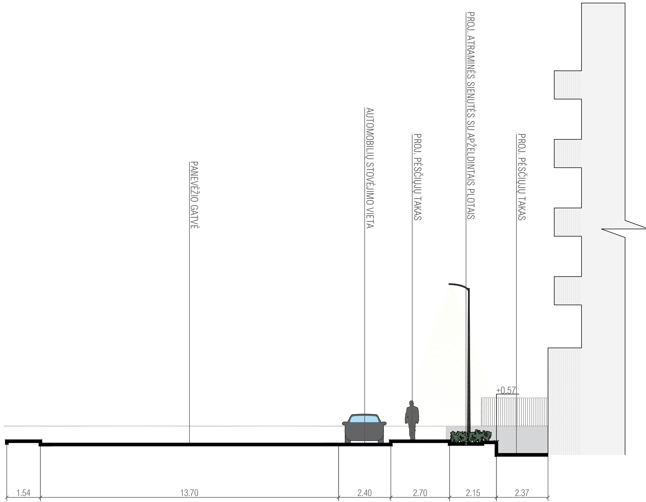
Pjūvis D-D
