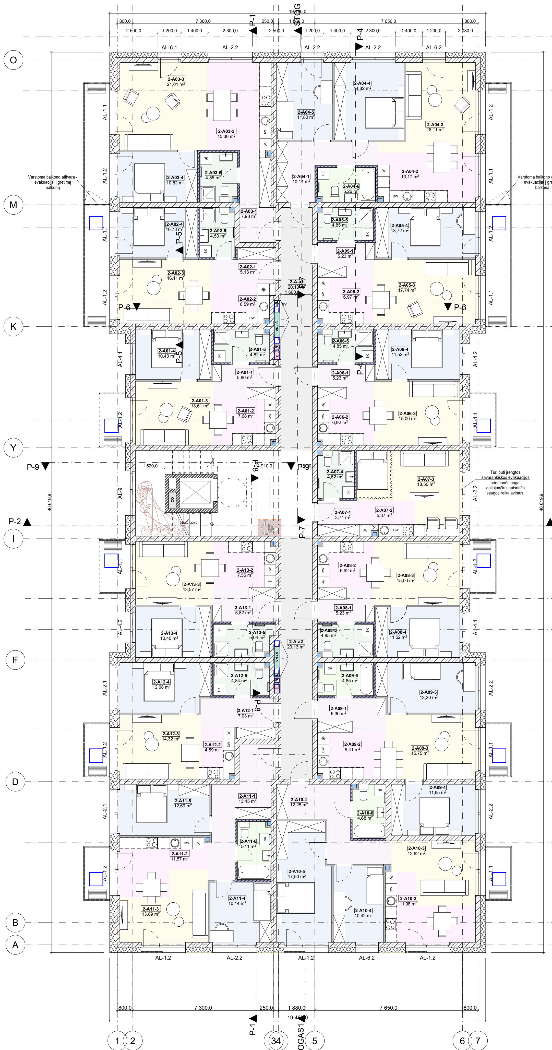
2 aukštas
