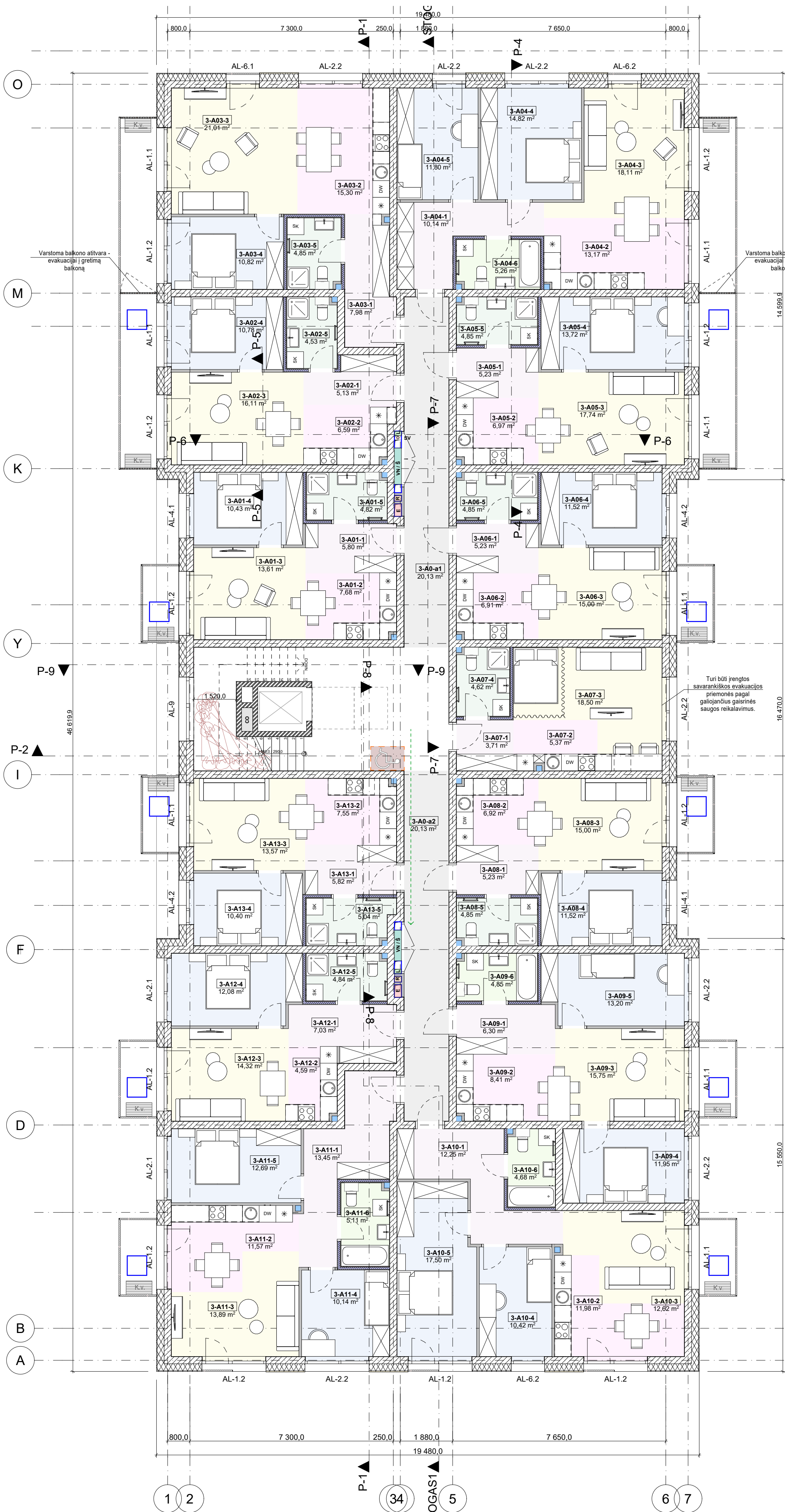
3 aukštas
