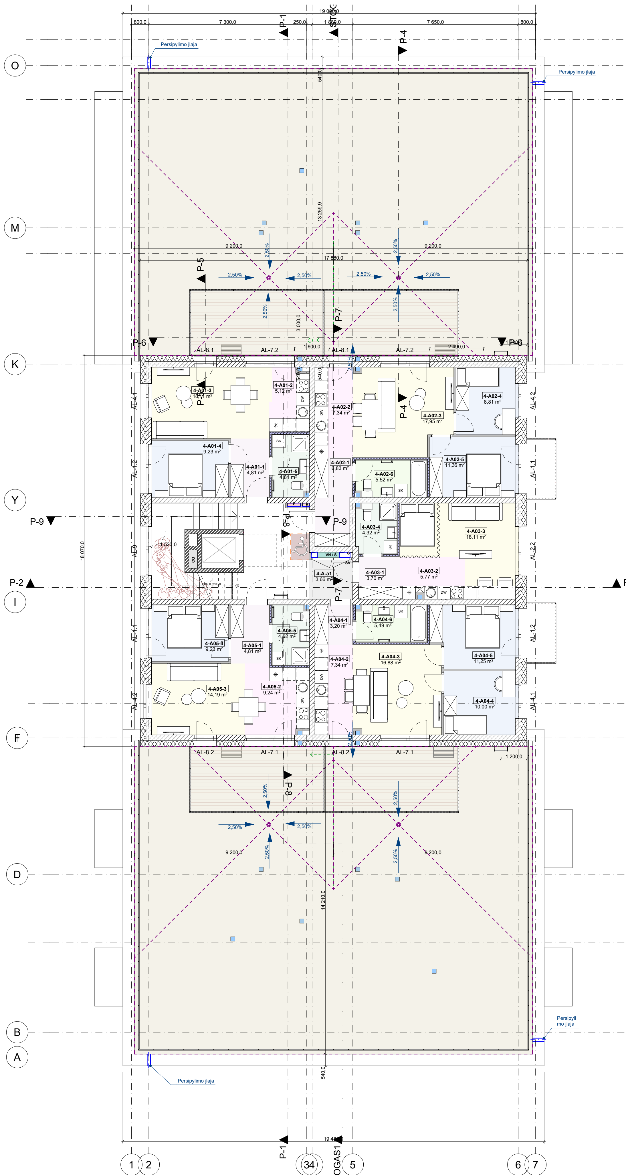
4 aukštas
