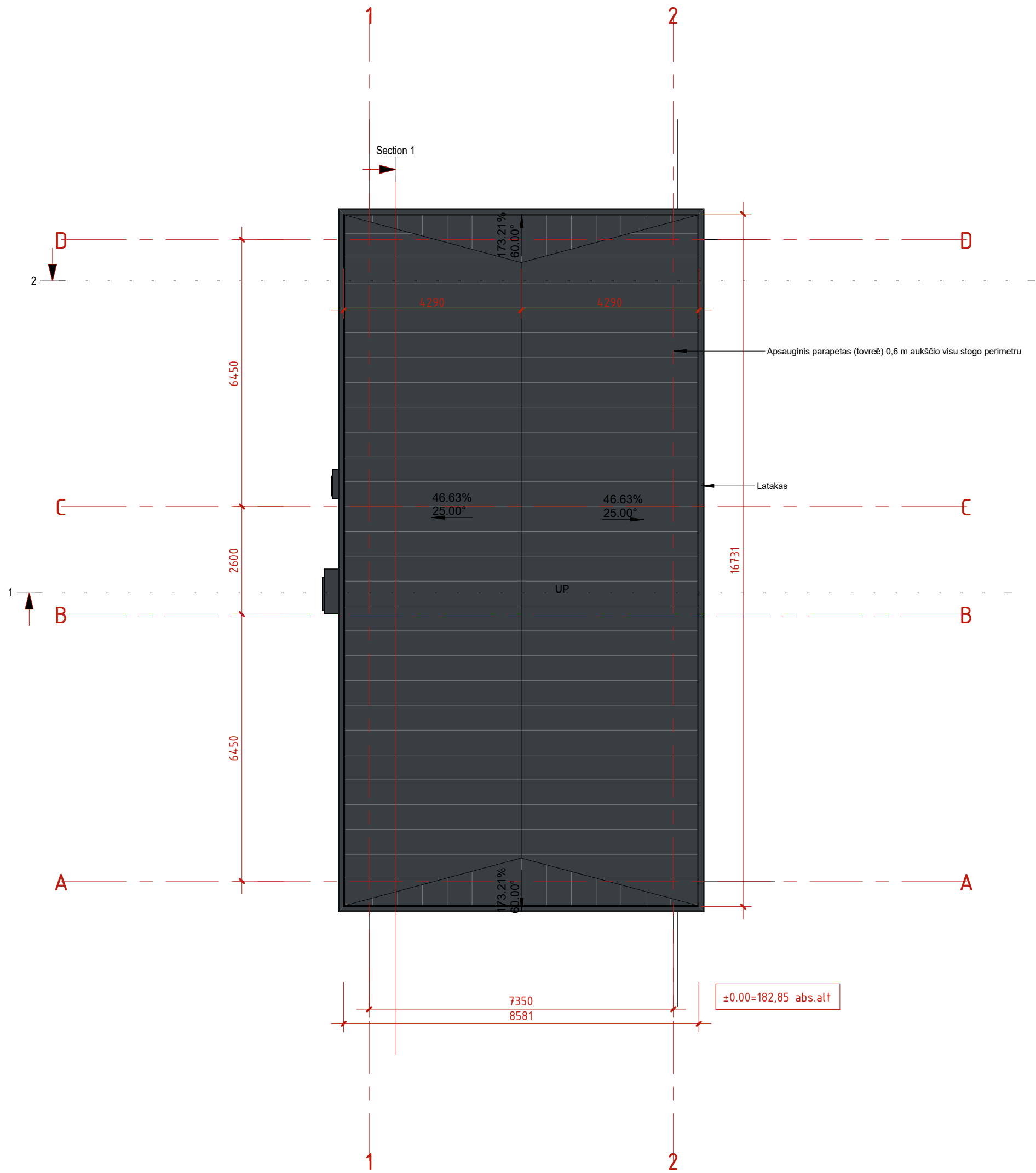
1 Stogo planas 1 : 100
