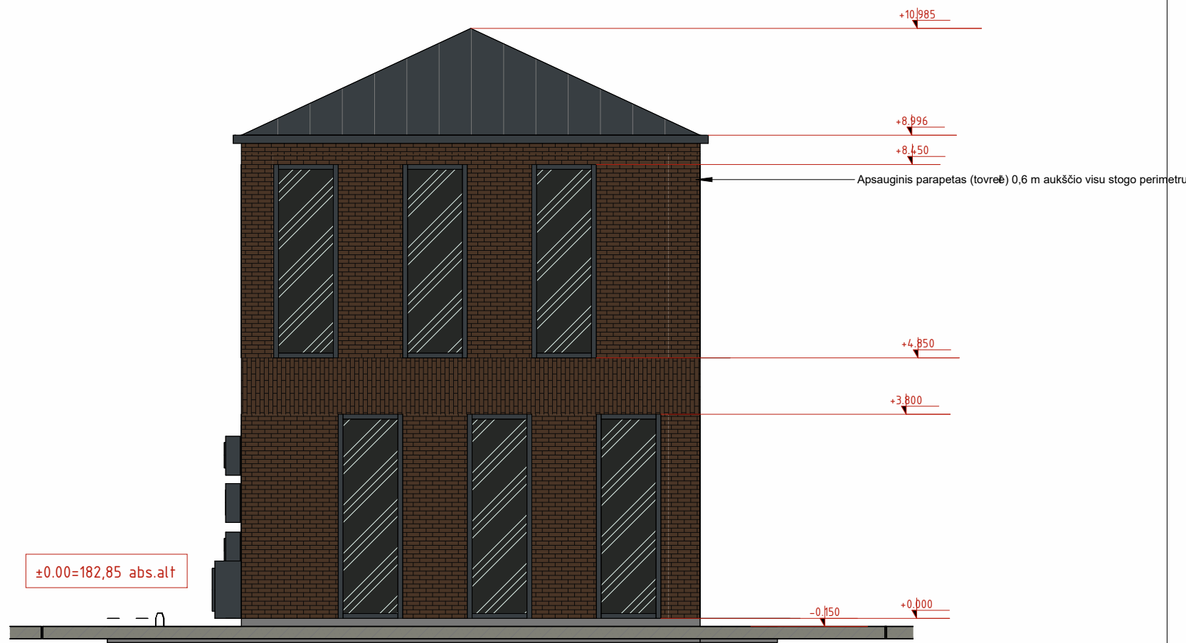
4 Fasadas 1-4 1 : 100
