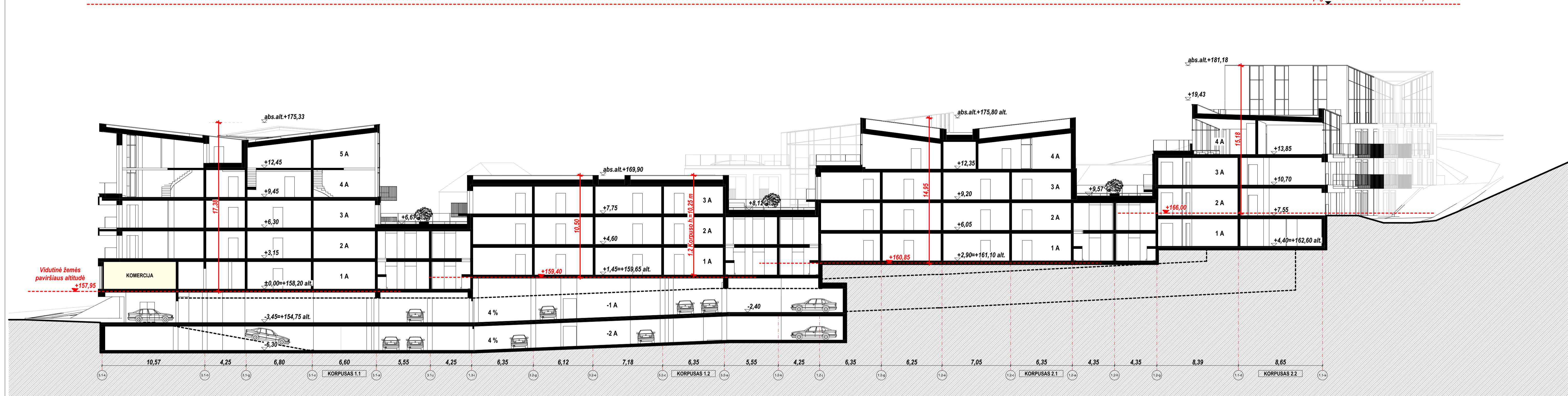
Išilginis pjūvis
