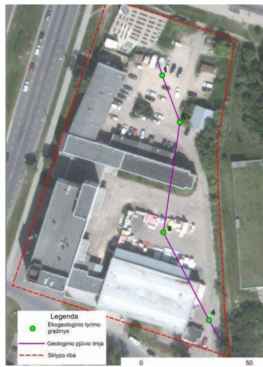
8 pav. Tiriamųjų gręžinių vietų išdėstymo schema
