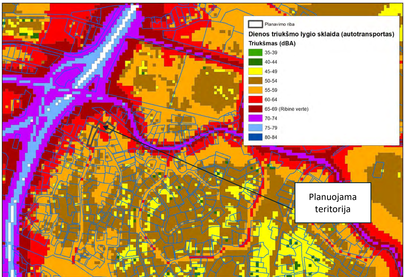
16 pav. Triukšmo sklaida nuo autotransporto dieną; ribinė vertė - 65 dBA
