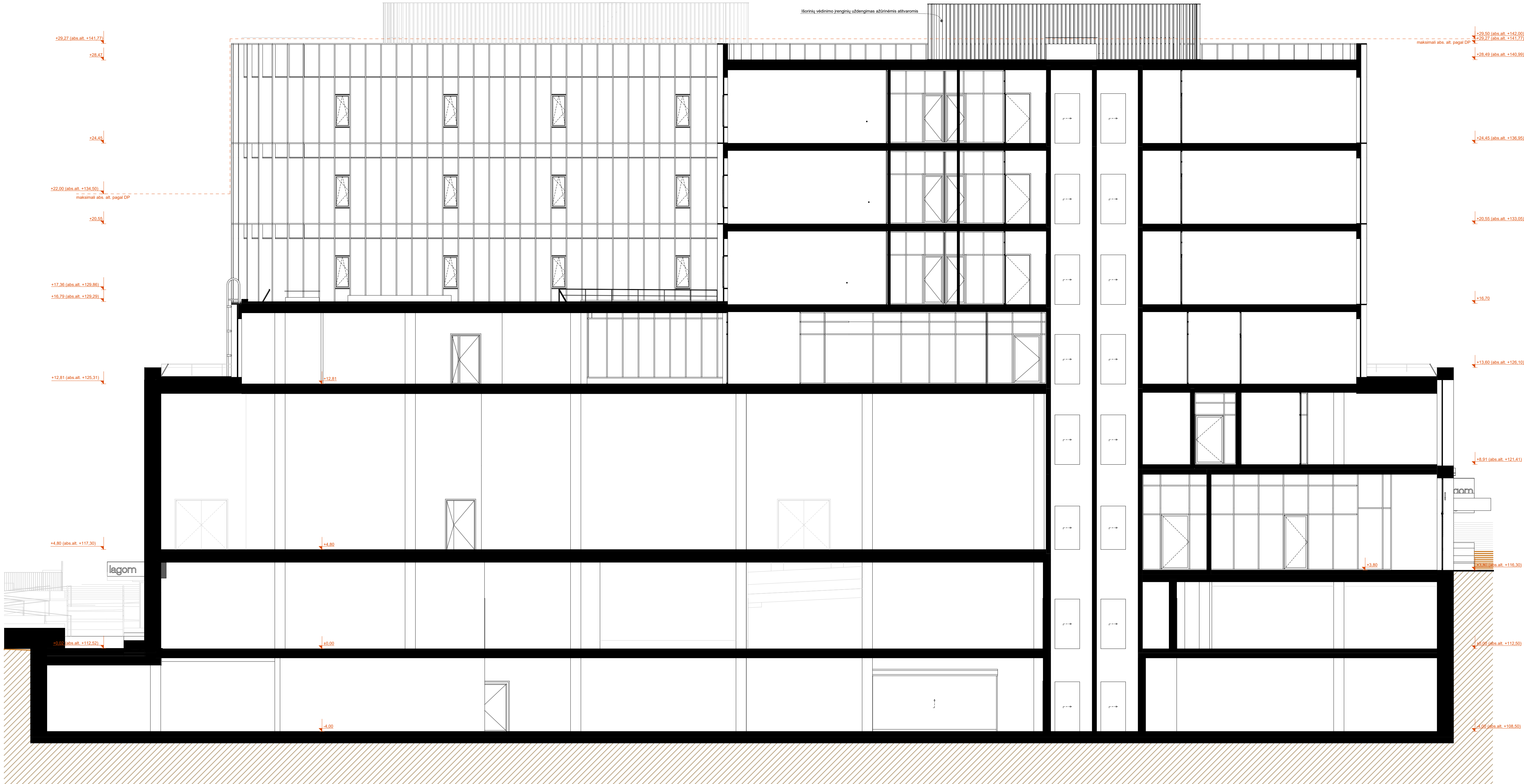
aP-6 Pjūvis 6 1:100
