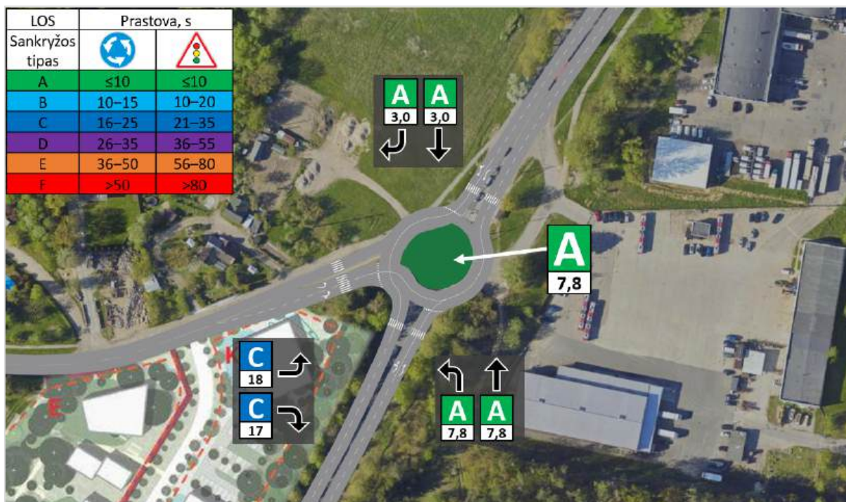
33 pav. Eismo kokybės lygis ir vidutinės prastovos sankryžoje Nr. 1, rytinis pikas Projektinis variantas Nr. 1 – žiedinė sankryža
