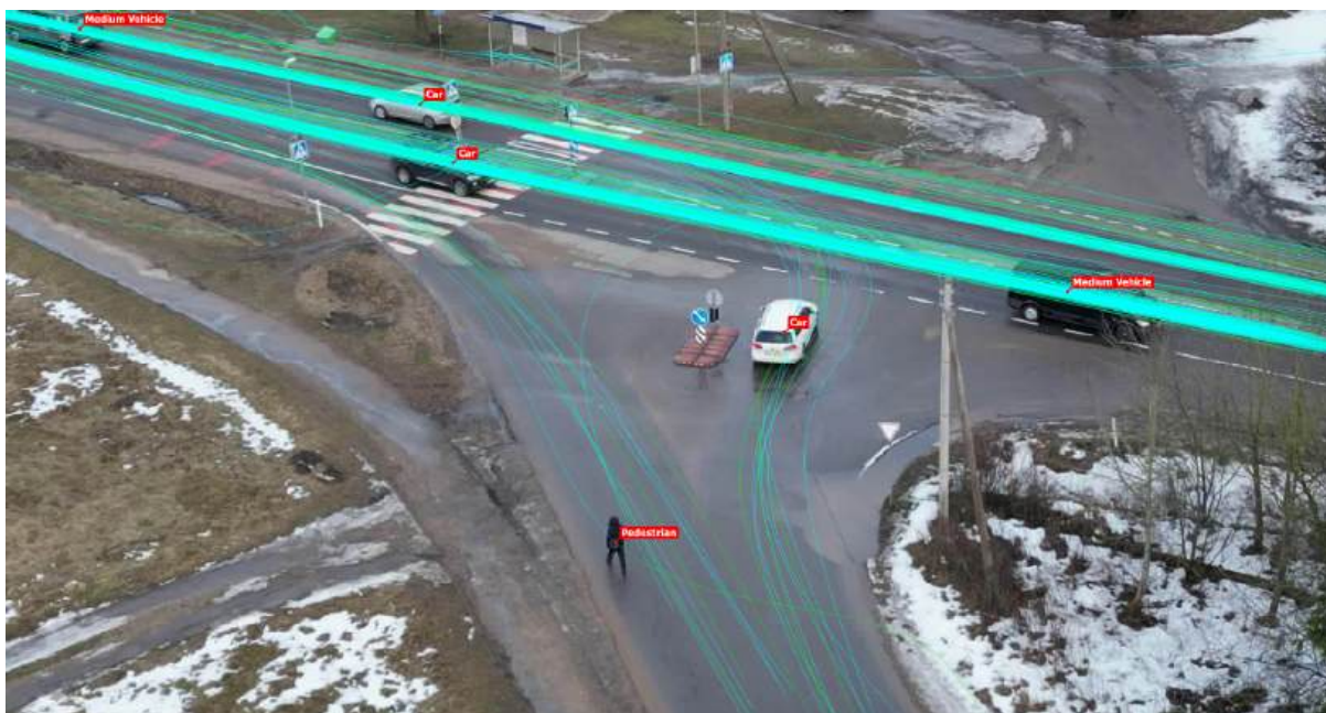
3 pav. Trumpalaikis tyrimas. Transporto priemonių judėjimo trajektorijos ir klasifikacija Eišiškių plento – Užusienio gatvės sankryža
