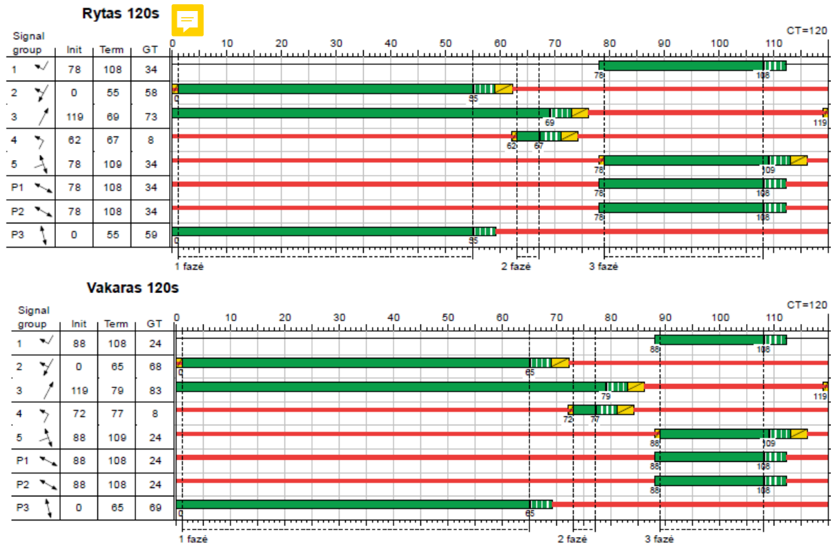
26 pav. Sankryža Nr. 1. Šviesoforų valdymo programos
