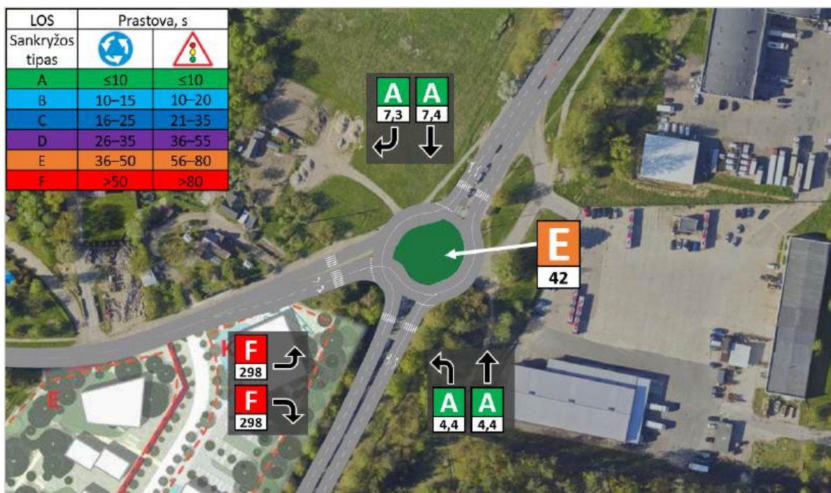
37 pav. Eismo kokybės lygis ir vidutinės prastovos sankryžoje Nr. 1, vakarinis pikas Projektinis variantas Nr. 1 – žiedinė sankryža
