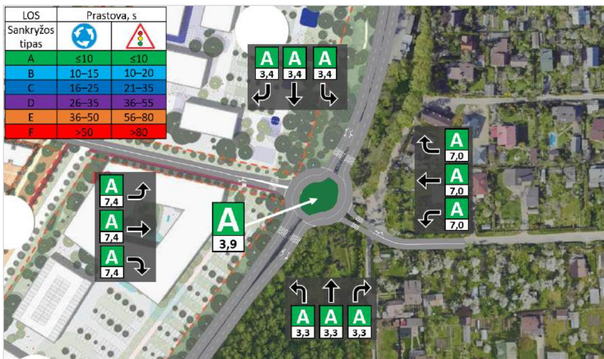
49 pav. Eismo kokybės lygis ir vidutinės prastovos sankryžoje Nr. 2, rytinis pikas Projektinis variantas Nr. 1 – žiedinė sankryža
