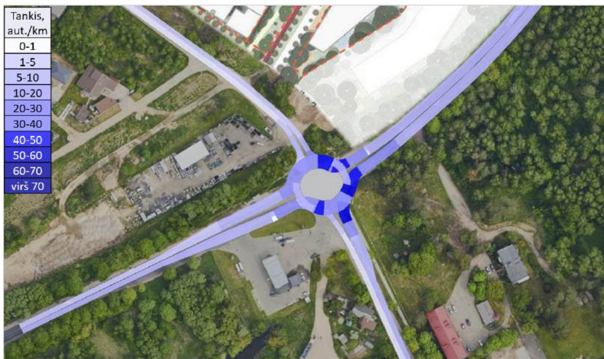
67 pav. Transporto priemonių tankis sankryžoje Nr. 3, rytinis pikas Projektinis variantas Nr. 1 – žiedinė sankryža
