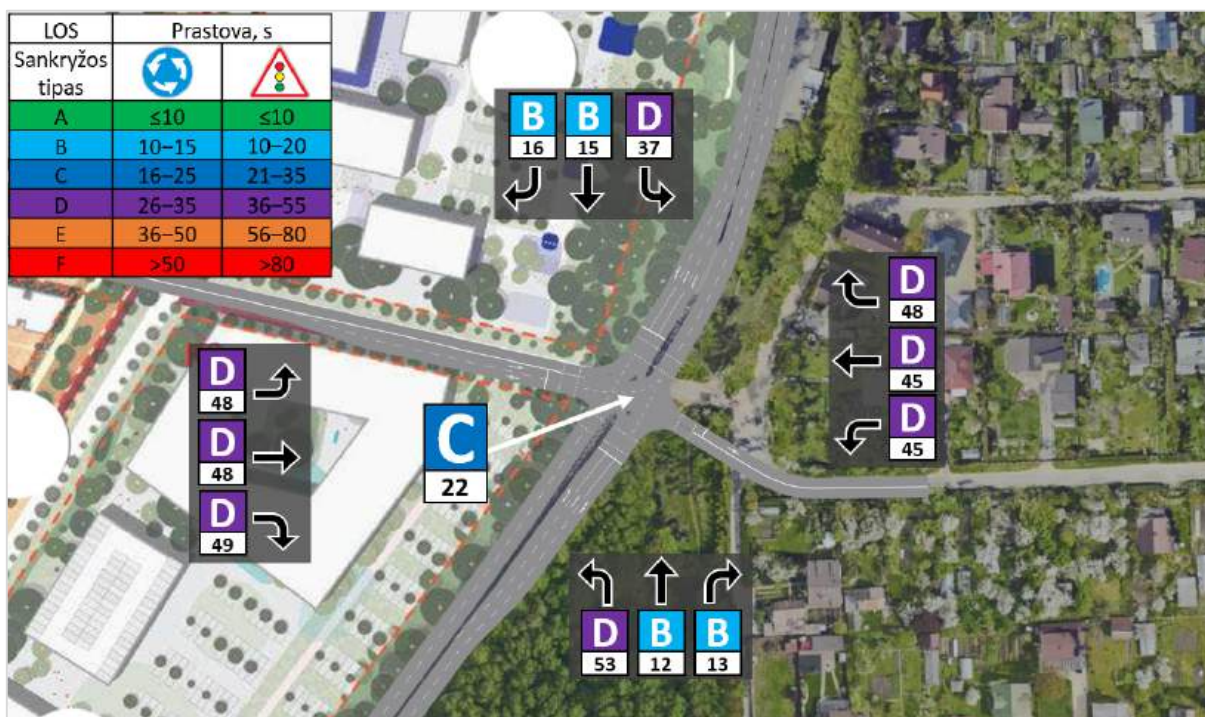
61 pav. Eismo kokybės lygis ir vidutinės prastovos sankryžoje Nr. 2, vakarinis pikas Projektinis variantas Nr. 2 – šviesoforinė sankryža
