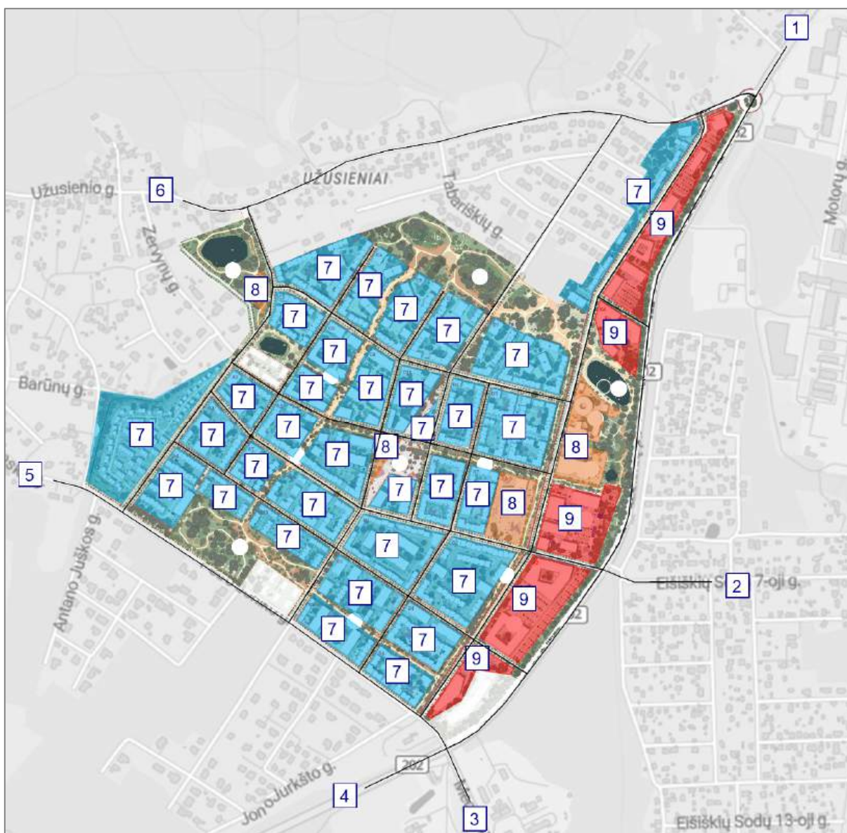
15 pav. Perspektyvinio scenarijaus transporto zonų schema. Viso 9 zonos
