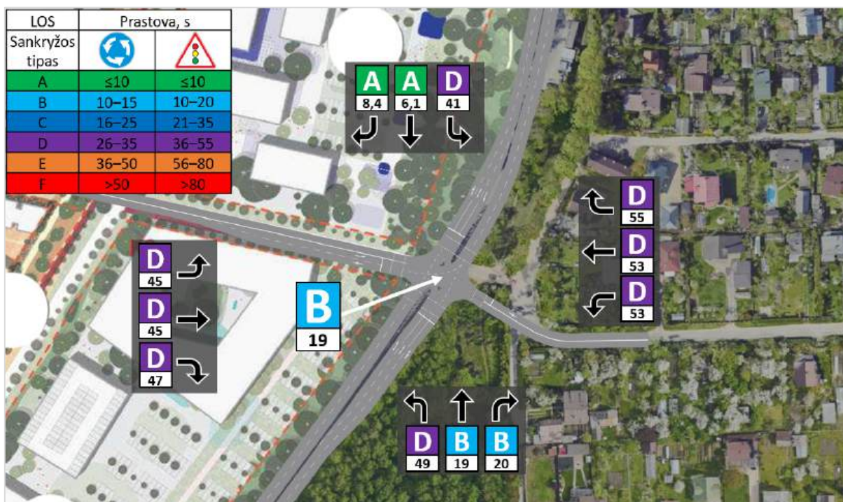
57 pav. Eismo kokybės lygis ir vidutinės prastovos sankryžoje Nr. 2, rytinis pikas Projektinis variantas Nr. 2 – šviesoforinė sankryža
