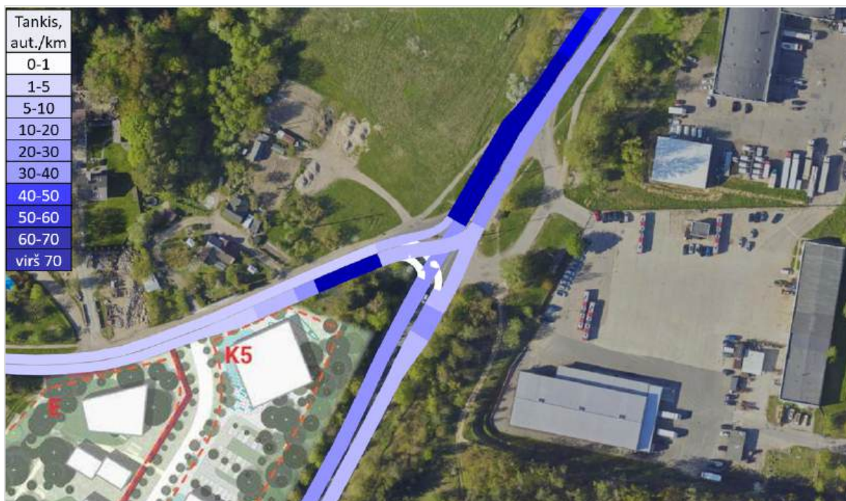
47 pav. Transporto priemonių tankis sankryžoje Nr. 1, vakarinis pikas Projektinis variantas Nr. 2 – šviesoforinė sankryža
