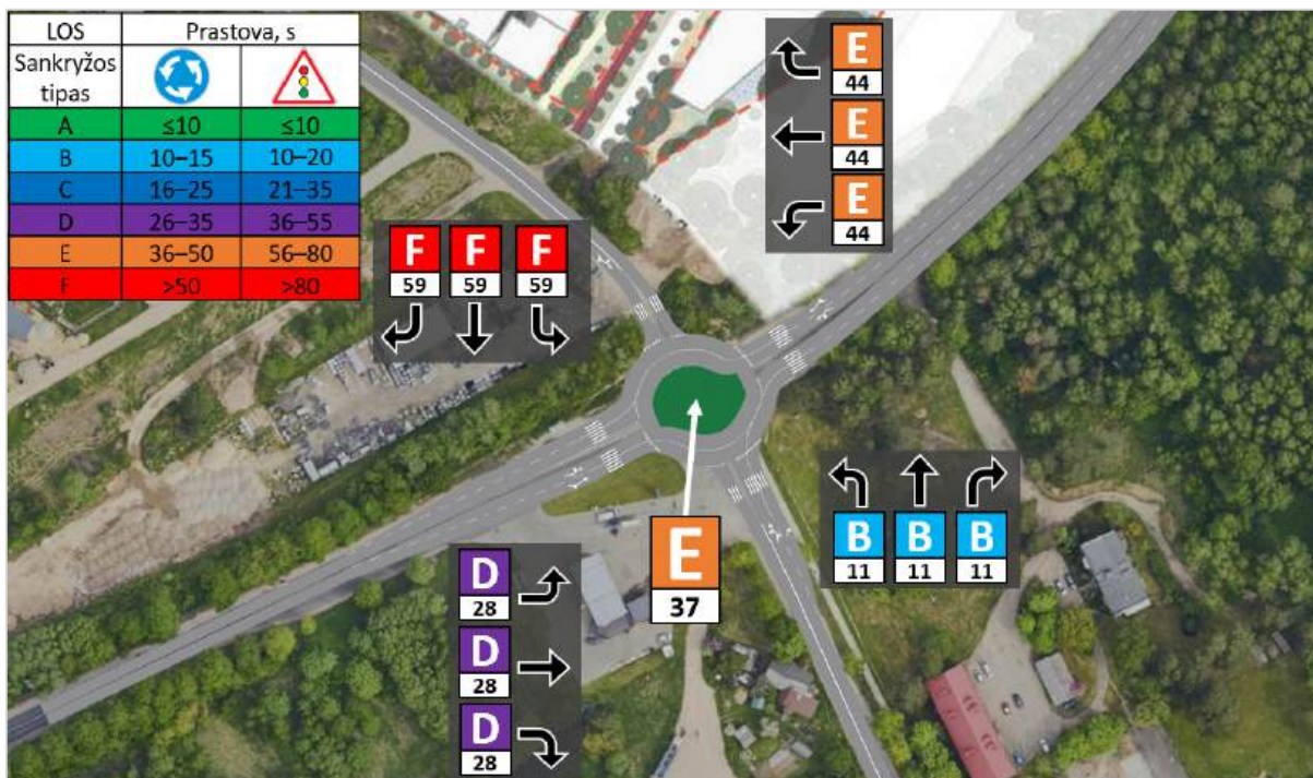
69 pav. Eismo kokybės lygis ir vidutinės prastovos sankryžoje Nr. 3, vakarinis pikas Projektinis variantas Nr. 1 – žiedinė sankryža
