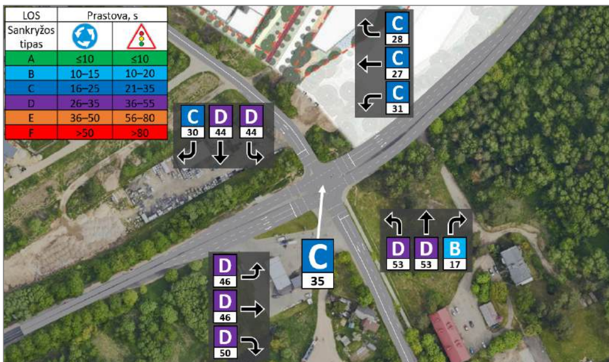
77 pav. Eismo kokybės lygis ir vidutinės prastovos sankryžoje Nr. 3, vakarinis pikas Projektinis variantas Nr. 2 – šviesoforinė sankryža
