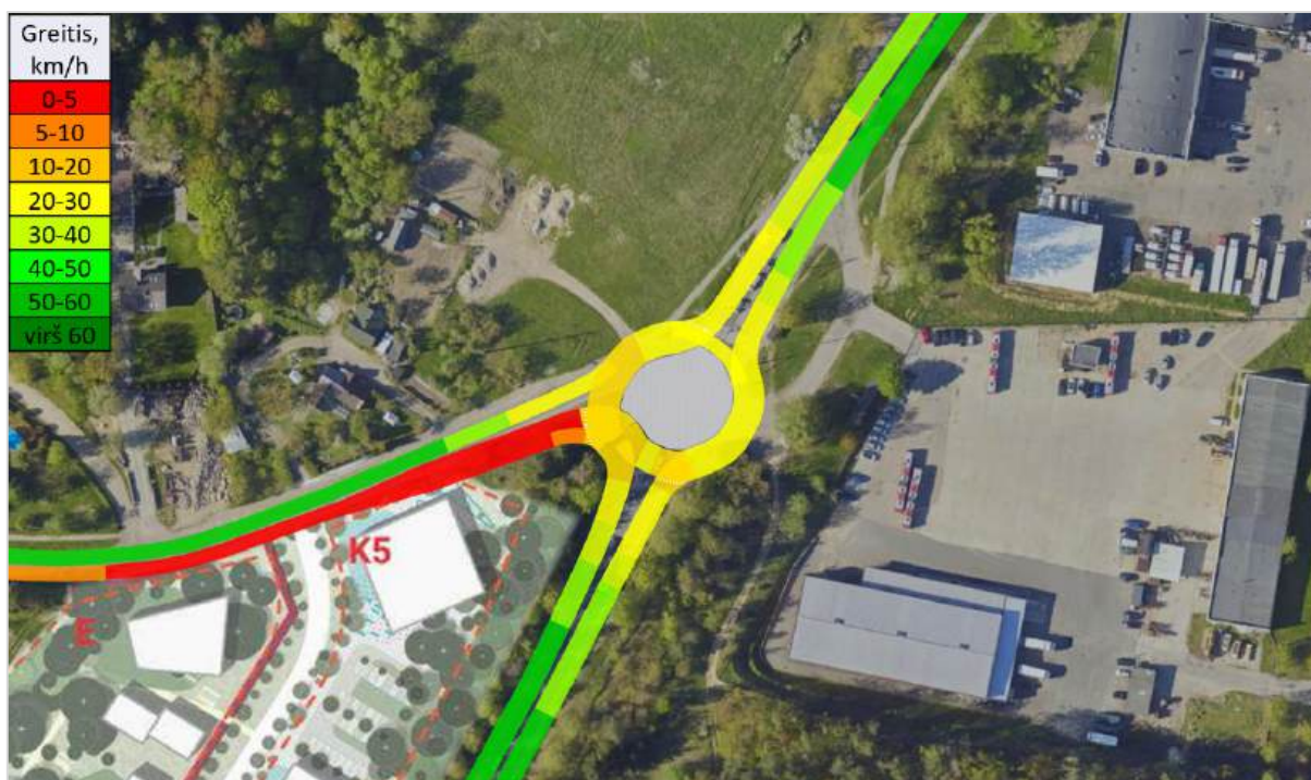
38 pav. Vidutinis automobilių greitis sankryžoje Nr. 1, vakarinis pikas Projektinis variantas Nr. 1 – žiedinė sankryža
