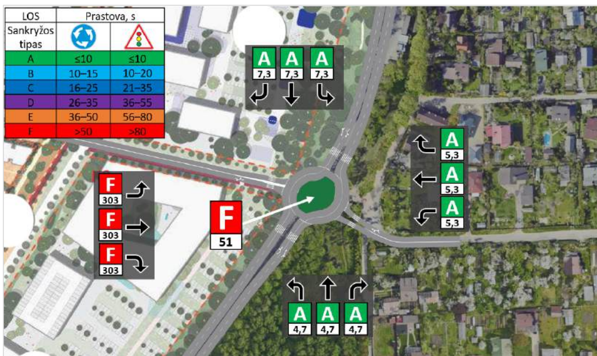
53 pav. Eismo kokybės lygis ir vidutinės prastovos sankryžoje Nr. 2, vakarinis pikas Projektinis variantas Nr. 1 – žiedinė sankryža
