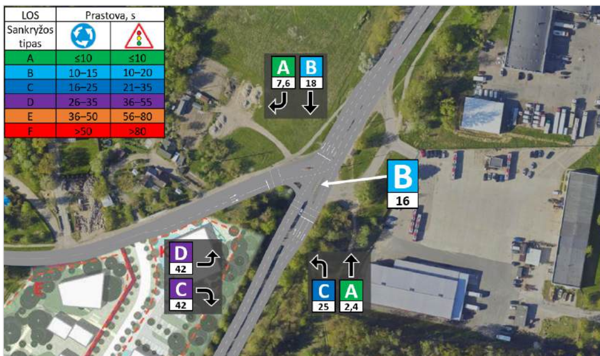
45 pav. Eismo kokybės lygis ir vidutinės prastovos sankryžoje Nr. 1, vakarinis pikas Projektinis variantas Nr. 2 – šviesoforinė sankryža
