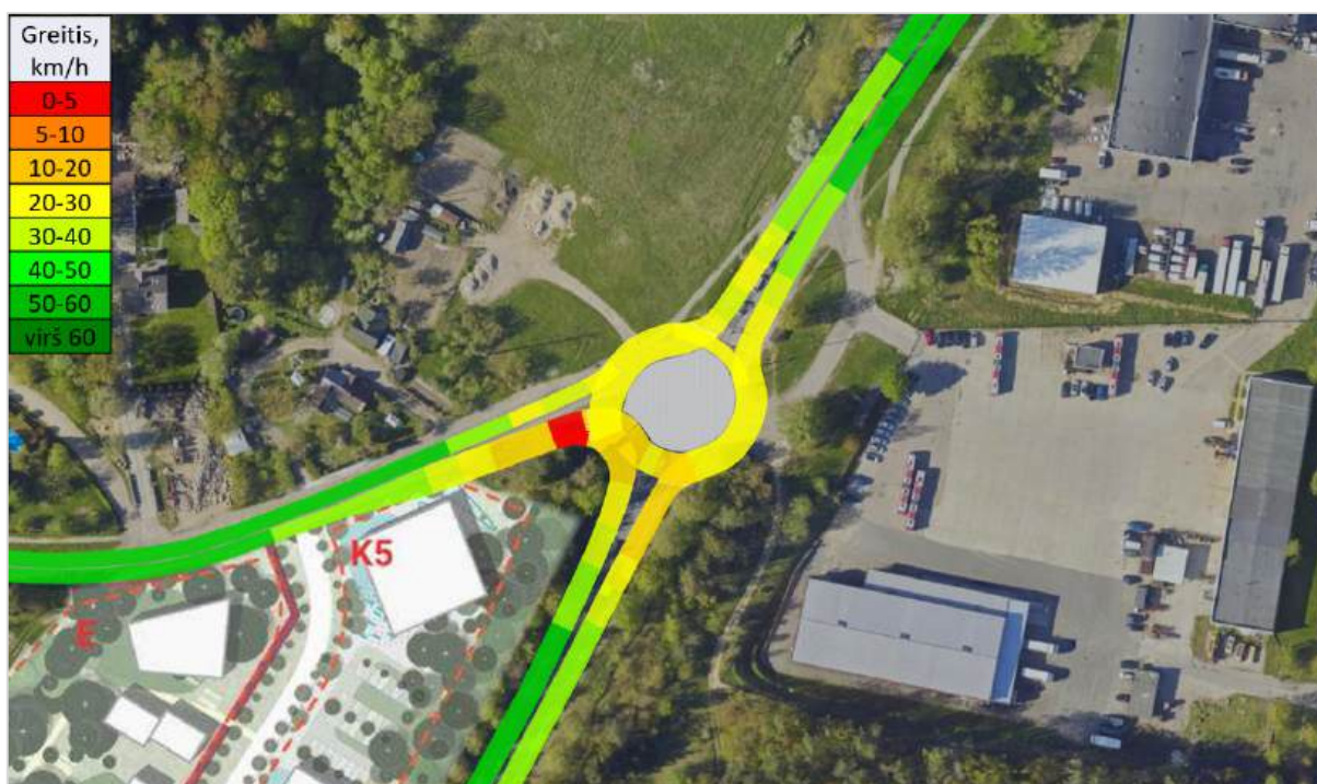
34 pav. Vidutinis automobilių greitis sankryžoje Nr. 1, rytinis pikas Projektinis variantas Nr. 1 – žiedinė sankryža
