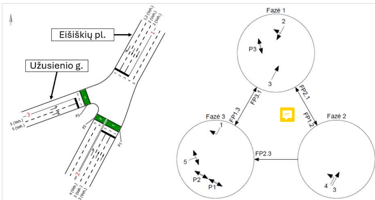
25 pav. Sankryža Nr. 1. Eišiškių pl. – Užušienio g.
