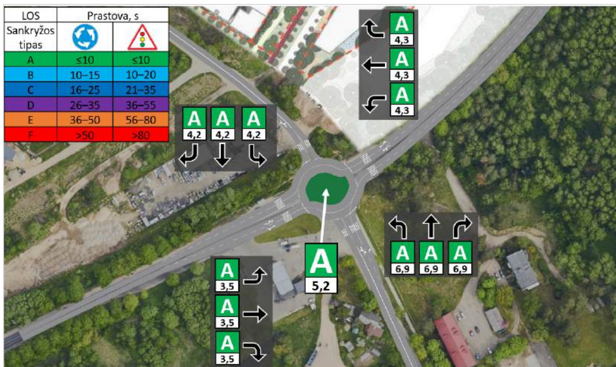
65 pav. Eismo kokybės lygis ir vidutinės prastovos sankryžoje Nr. 3, rytinis pikas Projektinis variantas Nr. 1 – žiedinė sankryža
