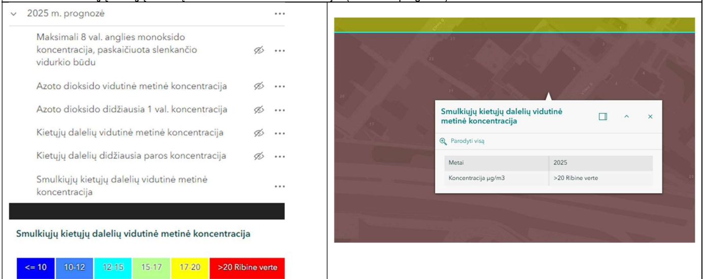
Pav. 48 Sieros dioksido vidutinė metinė koncentracija (2025 m. prognozė)
