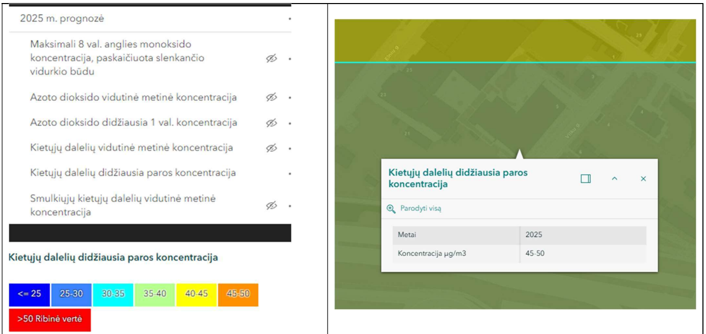
Pav. 47 Smulkiųjų kietųjų dalelių vidutinė metinė koncentracija (2025 m. prognozė).
