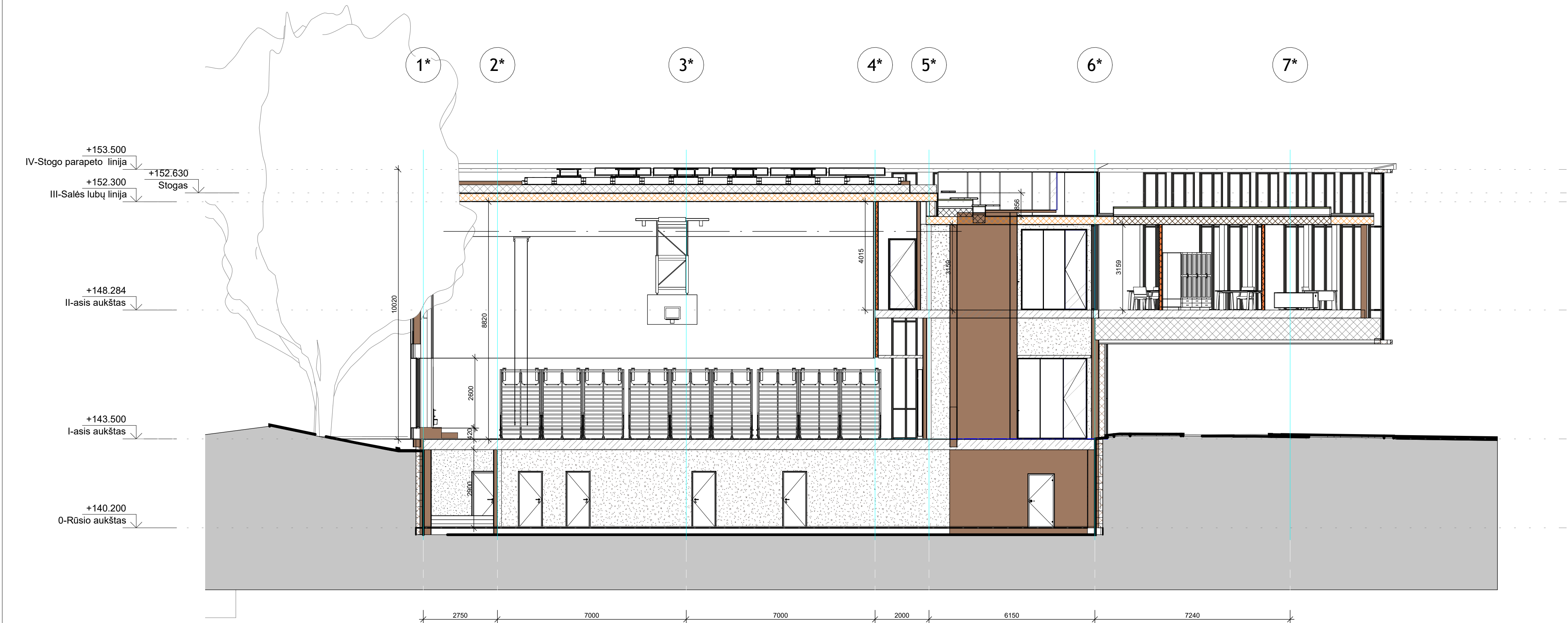
PJŪVIS - AA
