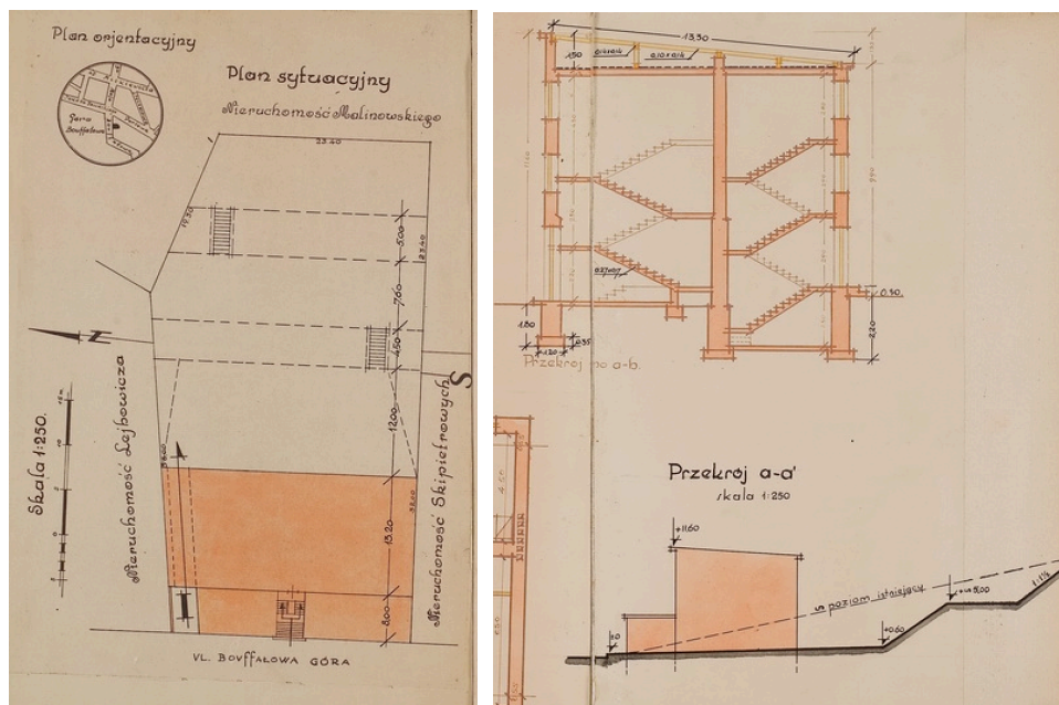
Sklypo planas ir namo pjūvis, M. S. Cholem, 1936 (neįgyvendintas), LCVA , f. 64, ap. 9, b. 2850, l. 1.
