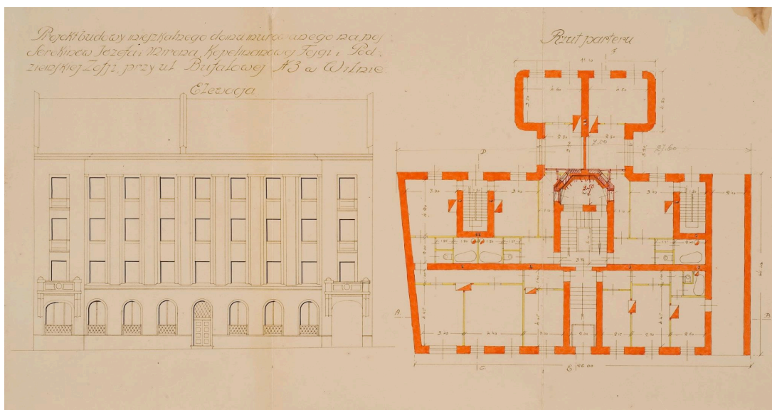
Jozefo ir Mirono Sorokinų, Fejgos Kopelman(owos) ir Zofijos Podziemskos daugiabučio namo statybos projektas (neįgyvendintas), archit. M. S. Cholem, 1928 m. LCVA , f. 64, ap. 9, b. 2850, l. 33.
