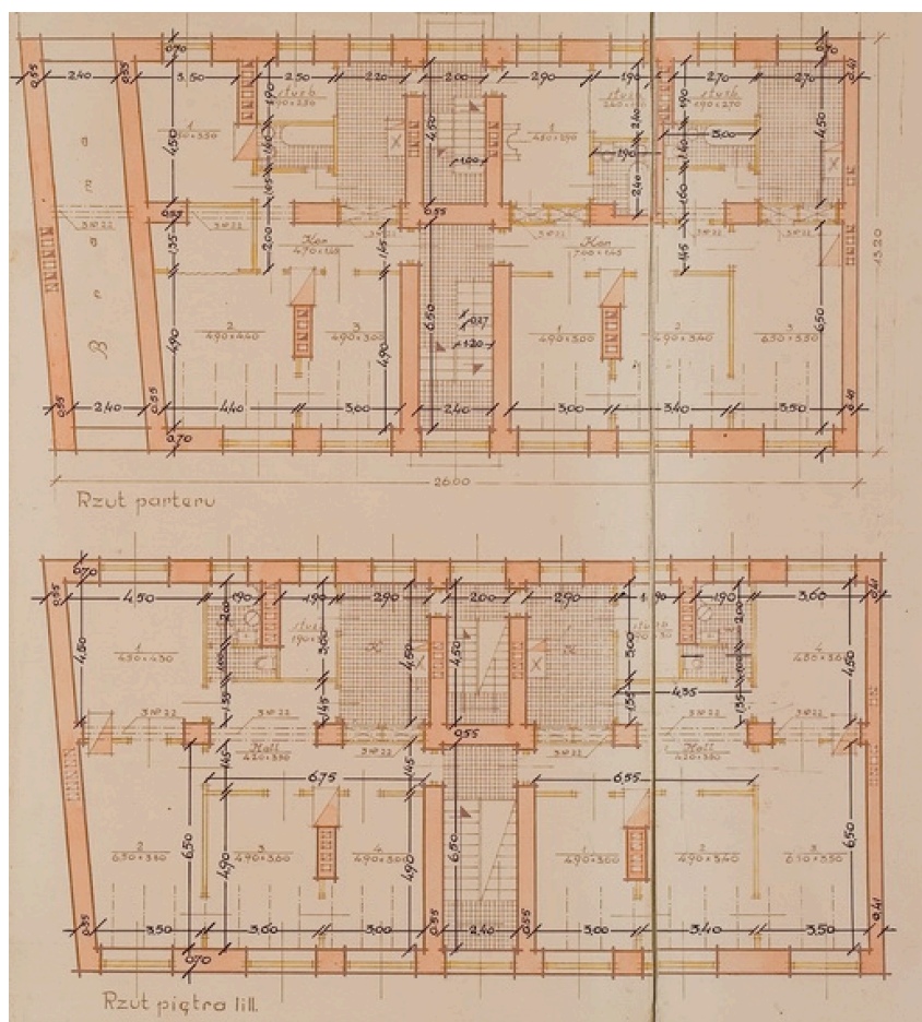
I (parter) ir II-III (piėtra) aukštų planai, M. S. Cholem, 1936 (neįgyvendintas), LCVA , f. 64, ap. 9, b. 2850, l. 1.
