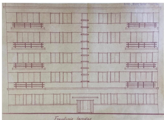
Abramo Strugaczio namo fasadas ir aukšto planas, A. Stulginskio g. 3, archit. M. S. Cholemas, VRVA , f. 761, ap. 4, b. 759.
