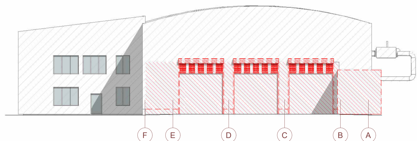
FASADAS F-A_DEMONTUOJAMA 1 : 200
