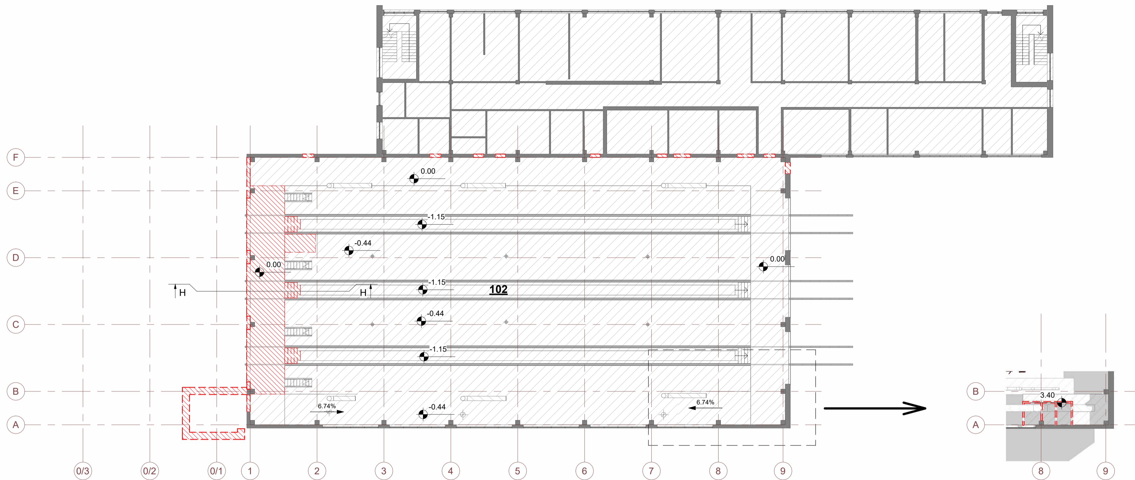
1_AUKŠTO DEMONTUOJAMŲ KONSTRUKCIJŲ PLANAS 1 : 200
