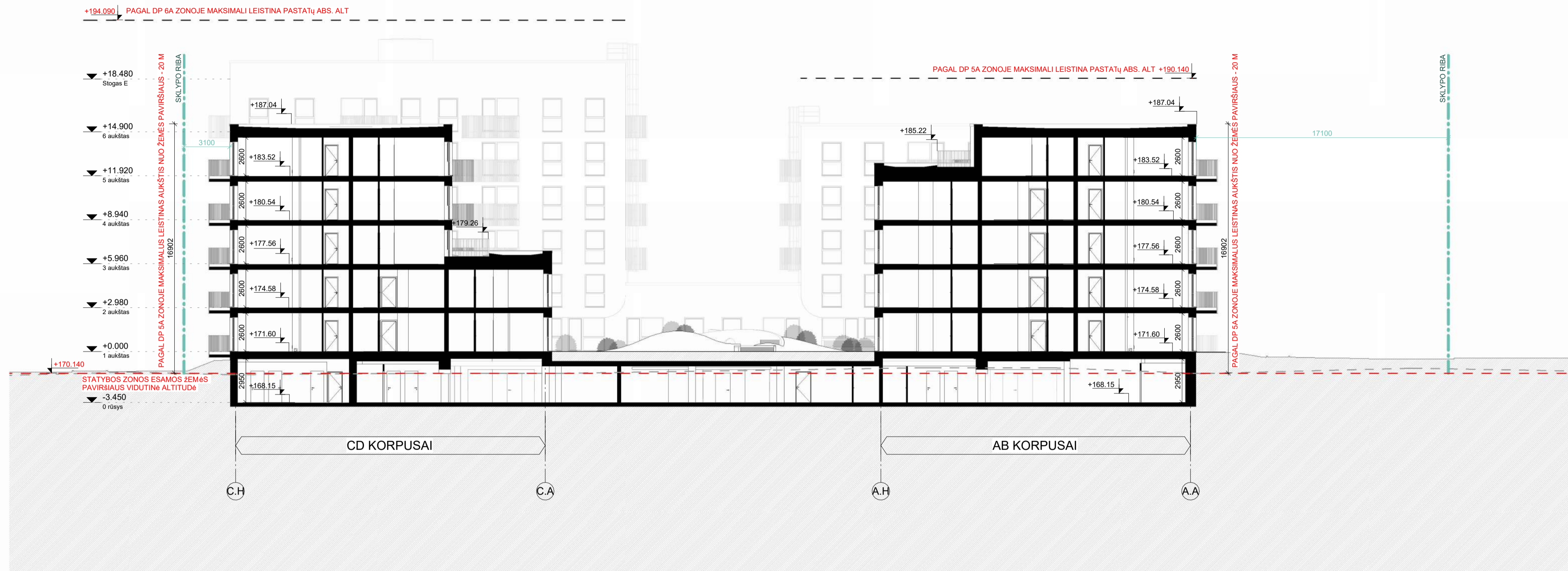
1. PJŪVIS 1-1 1:200
