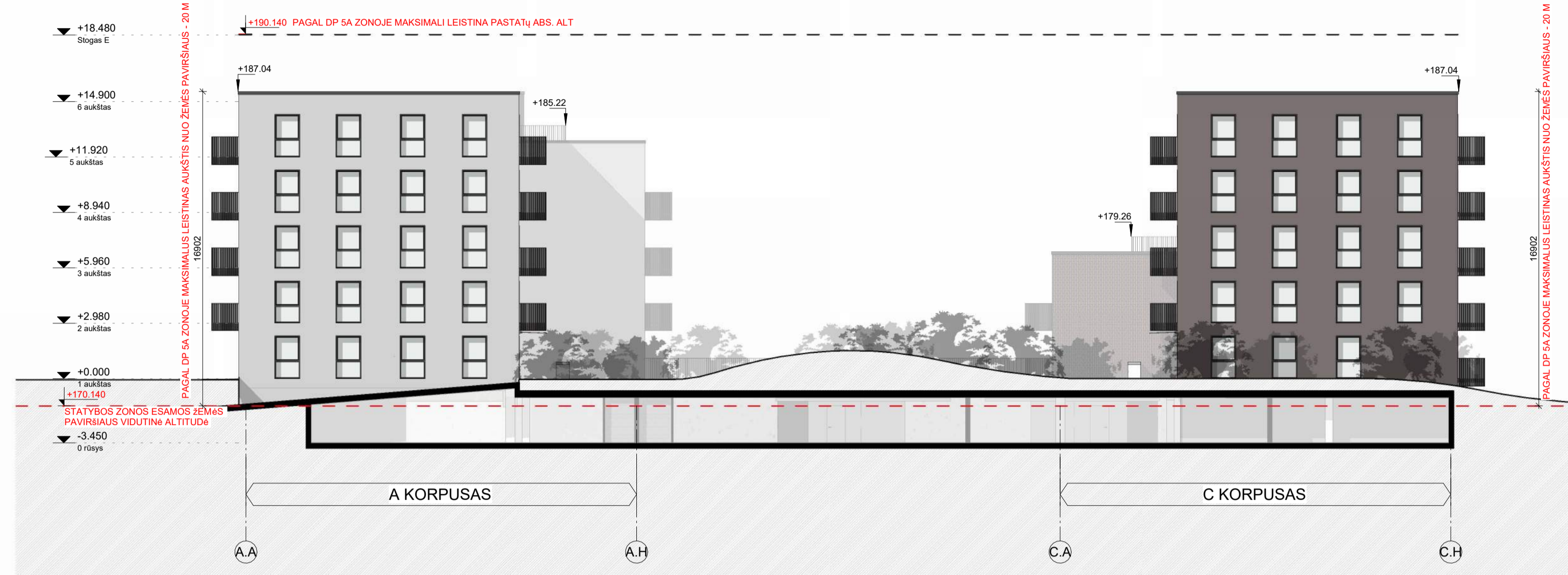
1. FASADAI TARP AŠIŲ A.A - C.H (KIEMO FASADAS)
