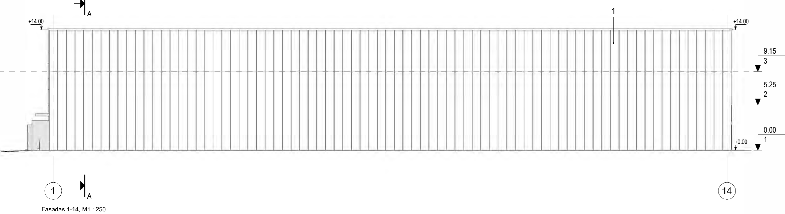
Fasadas 1-14, M1 : 250
