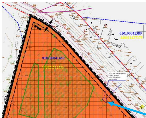
12 pav. Ištrauka iš rengiamo detaliojo plano pagrindinio brėžinio
